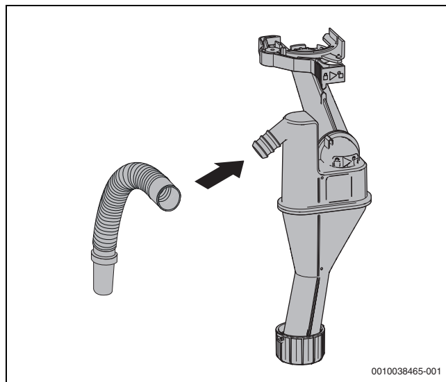
Мал. 30 Встановлення шланга для відведення конденсату на штуцер
