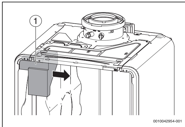
Мал. 28 Зняття пінопласту
