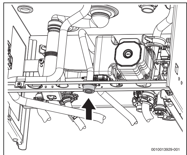
Мал. 23 Підключення зовнішнього мембранного компенсаційного бака
