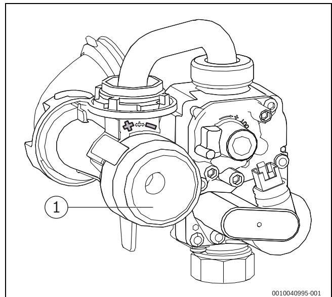
Мал. 38 Налаштування співвідношення газ-повітря
