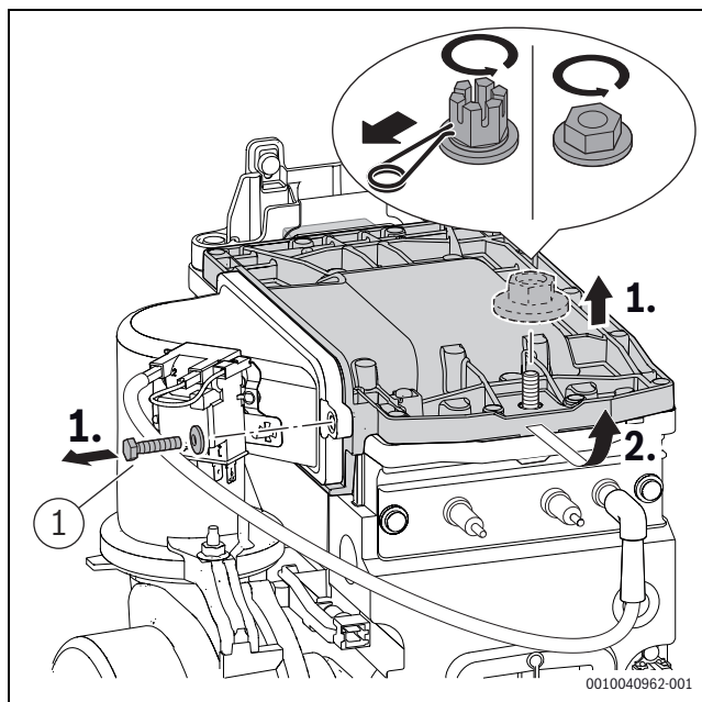
Мал. 45 Демонтаж кришки пальника
