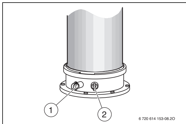
Мал. 42 Вимірювальний штуцер димових газів і штуцер для вимірювання повітря для горіння
