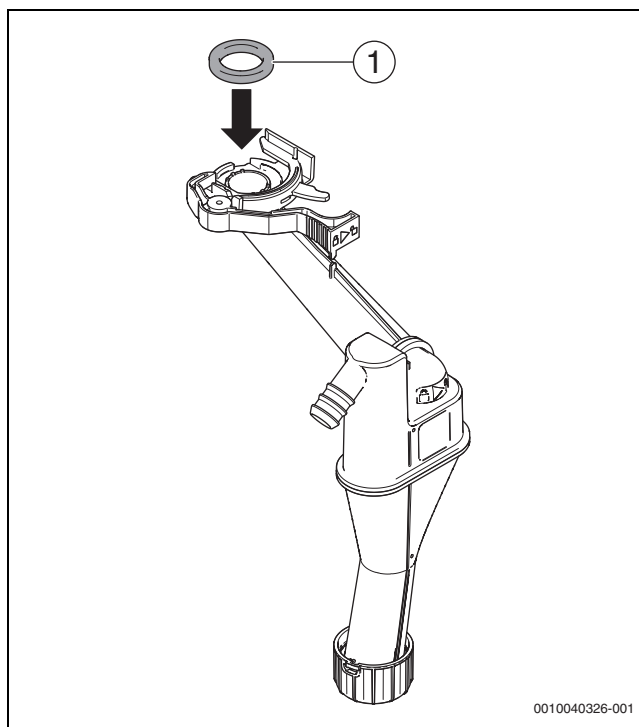
Мал. 52 Встановлення нового ущільнення на сифон для відведення конденсату
