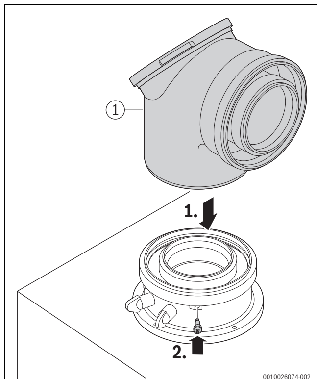
Мал. 32 Встановіть аксесуари для відведення відпрацьованих газів та зафіксуйте гвинтом
