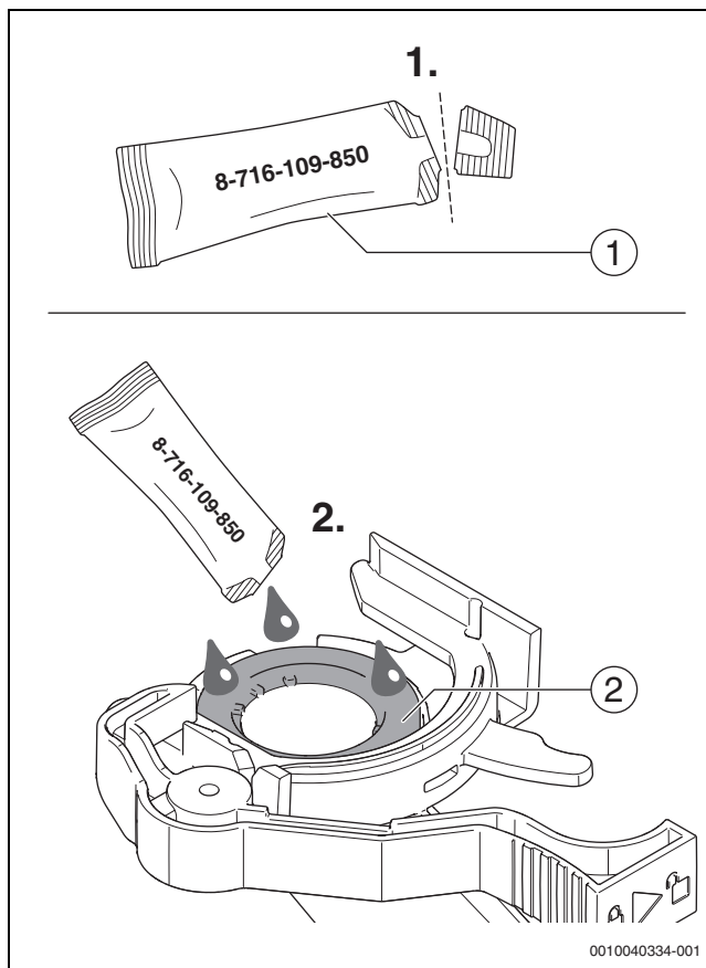
Мал. 53 Змащення ущільнення
