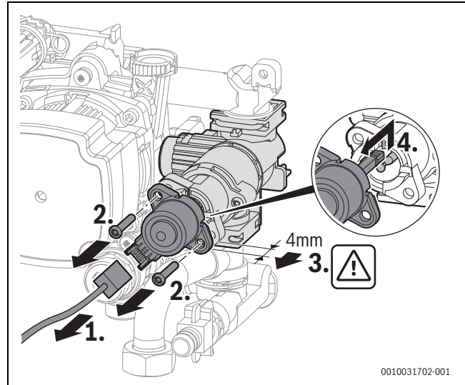
Мал. 57 Демонтаж двигуна 3-ходового клапана (варіант з гвинтами)
