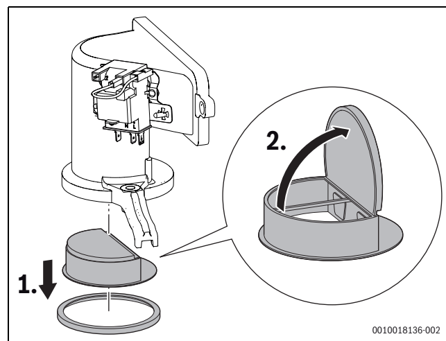
Мал. 49 Зворотний клапан змішувальної камери
