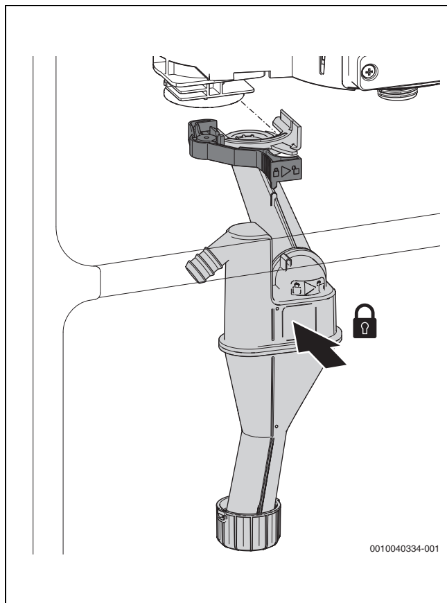
Мал. 54 Встановлення сифона для відведення конденсату
