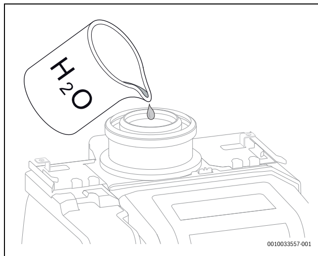
Мал. 31 Наповніть сифон для відведення конденсату водою
