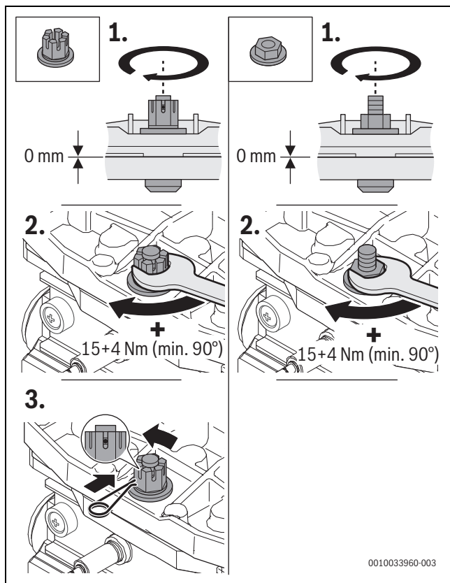
Мал. 47 Затягування гайки на кришці пальника
