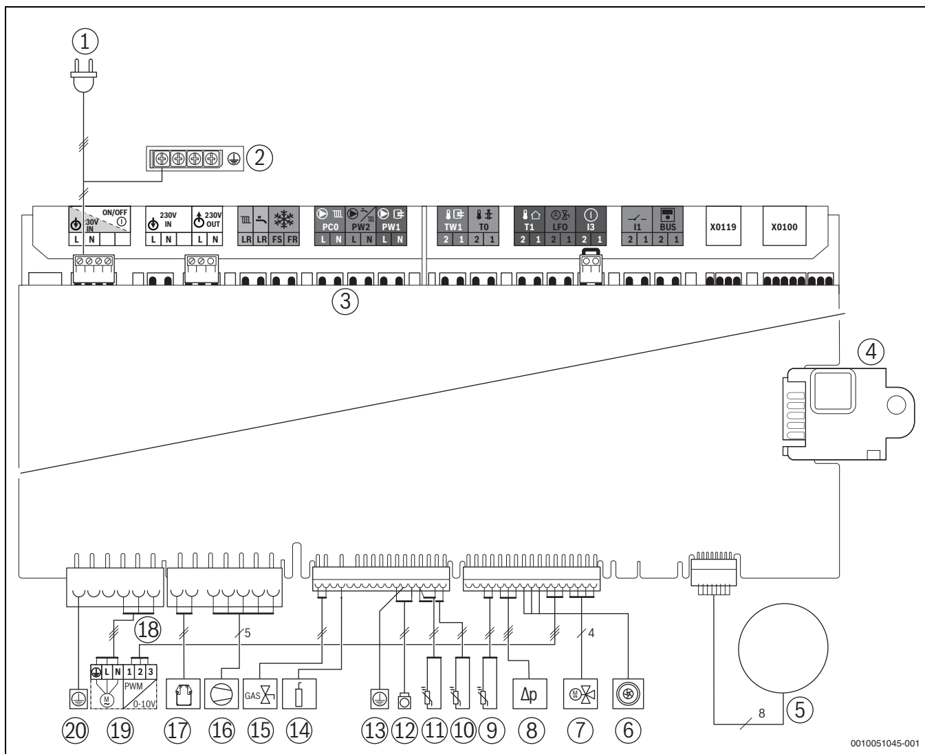
Мал. 60 Електричні підключення
