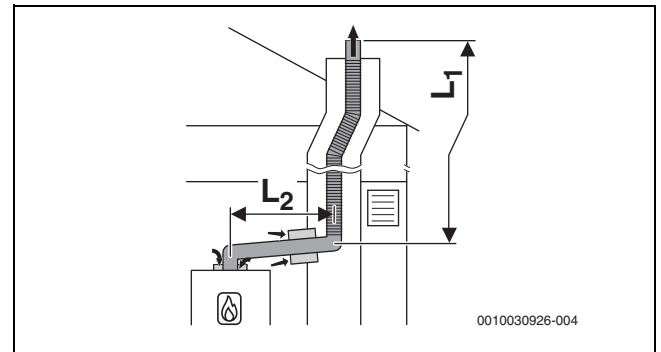
Мал. 19 Система відведення димових газів у шахті гнучкої конструкції відповідно до B 53p з подачею повітря у прилад з приміщення та концентричною з'єднувальною деталлю між котельним приміщенням та шахтою
