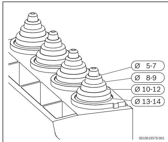
Мал. 34 Підгонка фіксатора проводу до діаметра кабелю
