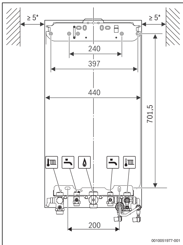
Мал. 3 Вид спереду (мм) з монтажною приєднувальною панеллю (додаткові комплектуючі)
