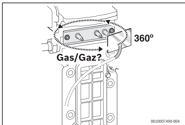
Мал. 44 Перевірка герметичності
