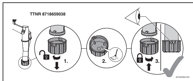
Мал. 51 Очищення брудовловлювача
