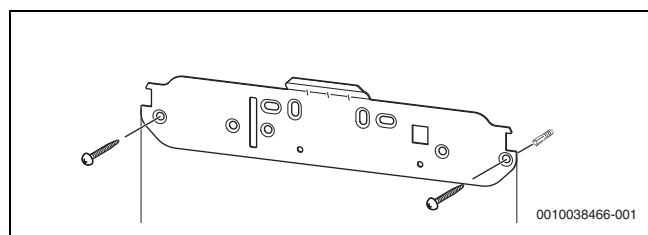
Мал. 26 Монтаж монтажної планки
