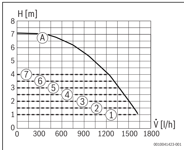
Мал. 59 Характеристики насоса та криві характеристик насоса
