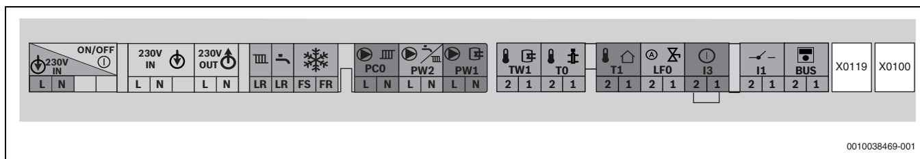
Мал. 35 Клемна колодка для зовнішньої системи керування
