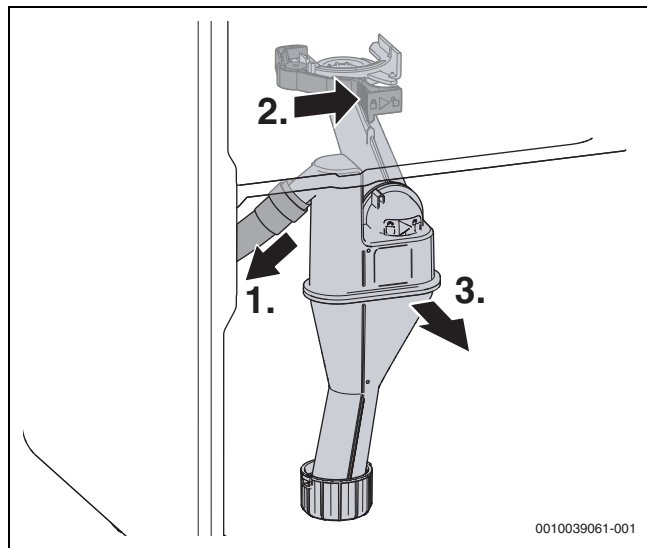
Мал. 50 Демонтаж сифона для конденсату
