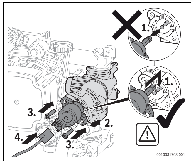
Мал. 58 Монтаж двигуна 3-ходового клапана (варіант з гвинтами)
