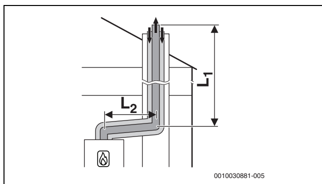
Мал. 11 Концентрична система транспортування повітря для горіння та димових газів згідно з C 33x у шахті
