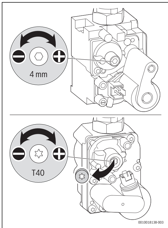
Мал. 40 Налаштування вмісту CO 2 або O 2
