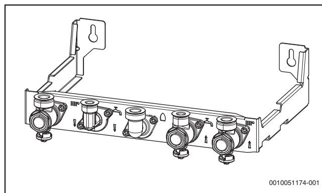
Мал. 27 Монтаж труб з ущільненнями на монтажну приєднувальну панель
