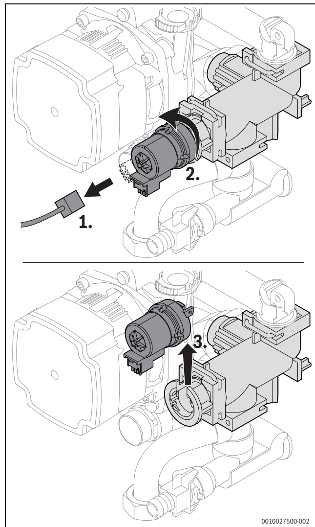
Мал. 55 Демонтаж двигуна 3-ходового клапана (варіант без гвинтів)
