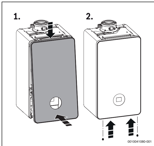
Мал. 36 Монтаж кожуха
