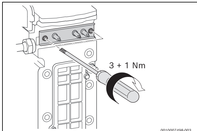
Мал. 43 Монтаж набору електродів
